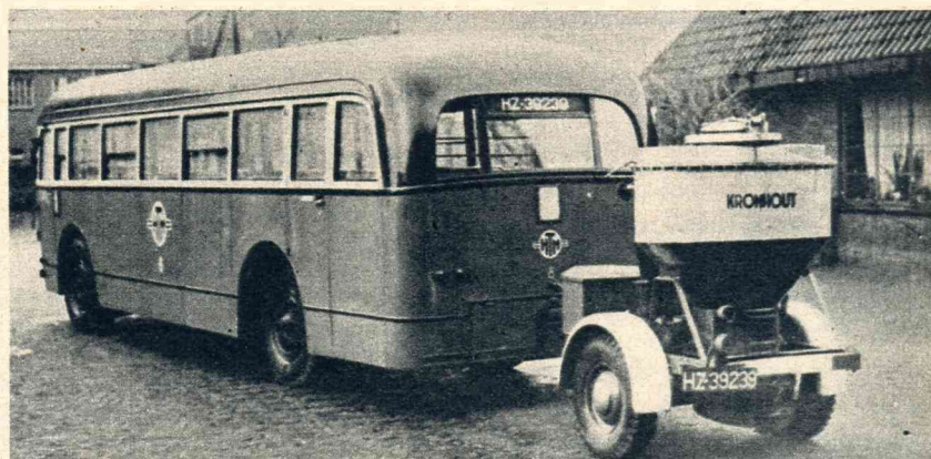
Ook de bussen van de H.T.M. te Den Haag zullen in den vervolge op houtgas gaan loopen. Het eerste exemplaar is afgeleverd en heeft met succes zijn proefrit afgelegd.
