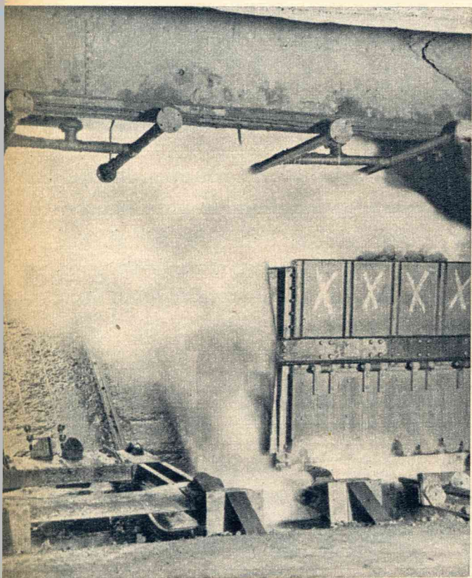
Een sissende wolk is het gevolg van het doovende water op de witgloeiende cokes. De foto toont de bluschinrichting, links ziet men het wagentje, waarop de bak na het blussen langs een helling naar boven gebracht wordt.
