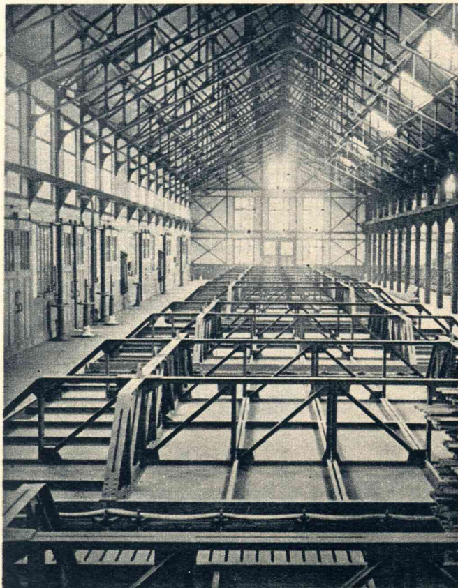
Het hangspoor, een zg. „Telpherbaan”, met opslagplaats van de naar stukgrootte gesorteerde cokes.
