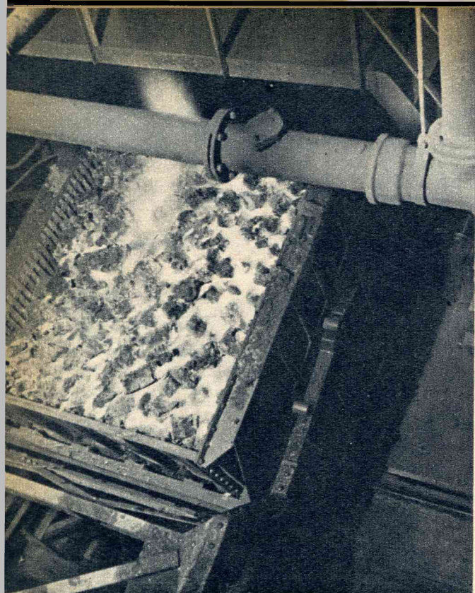
Witgloeiende bak cokes op weg naar de bluschinrichting.
