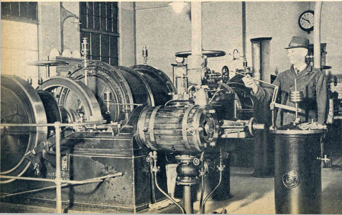
De zg. „exhausters”, door een stoommachine aangedreven gaspompen, die het gas uit de stokerij aanzuigen en het door de verschillende volgende zuiveringsstoestellen naar den gashouder persen.
