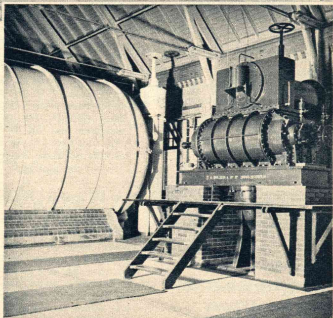
De gasmeter, waarmee van uur tot uur de hoeveelheid wordt vastgesteld van het in de stokerij gemaakte steenkolengas.
