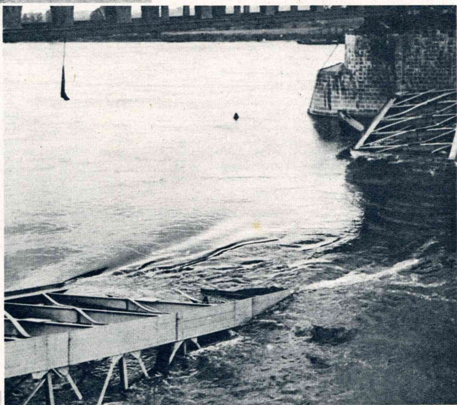
Bij de pogingen om een der overspanningen van de brug te Zaltbommel naar Hedel te vervoeren is deze gekanteld en op de vier drijvende bokken terechtgekomen, die er onder lagen. Zeven arbeiders werden gedood en velen gewond.
