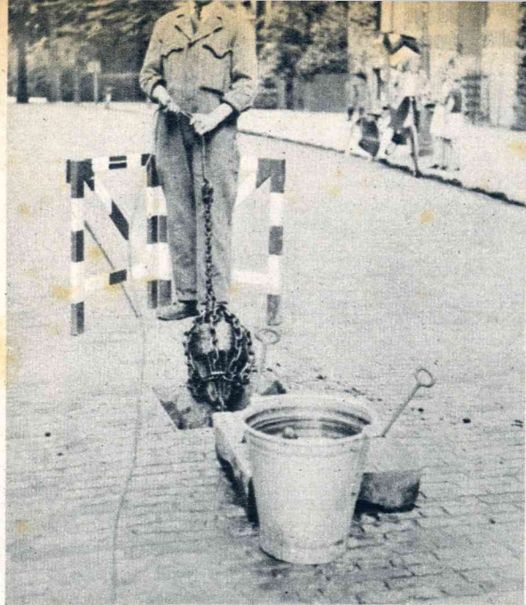
Nadat eerst met buigzame rieten staven de verbinding tusschen twee putten verkregen is, laat een man „de kat” in den put zakken. Dit is een ijzeren bol, omwonden met ijzeren kettingen, die door de rioolbuis getrokken wordt en het slib voor zich uit wegveegt.
