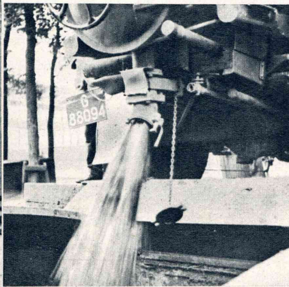
Een der kolossale nieuwe putzuigmachines stort zijn viezen last in een der schuiten van de Stadsreiniging, welke hygiënisch overdekt in de grachten liggen en het verzamelde slib naar de buiten de stad gelegen baggerbergplaatsen brengen.
