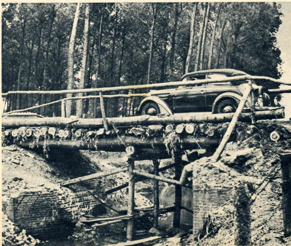
Een noodbruggetje in Noord-Brabant.
