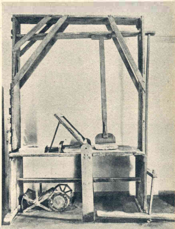
Eerste drukpers voor steendruk.
