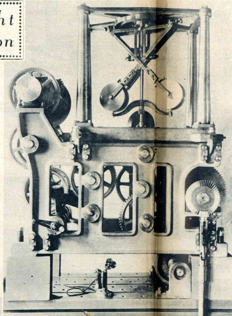
Deze groote machine is niets dan een uurwerk, ongeveer geconstrueerd als een gewoon horloge. Zij richt de beweging van den telescoop naar den loop van de sterren. Naar de grootte van de telefoon kan men de afmetingen beoordeelen.
