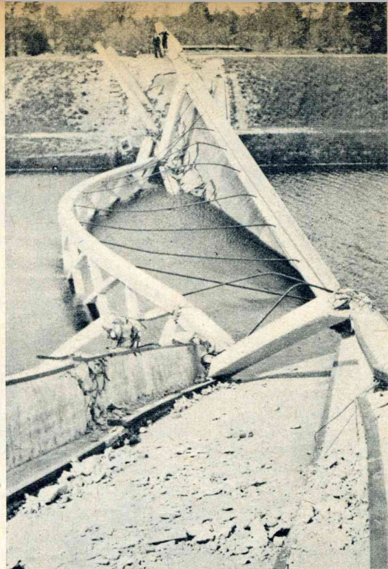
De brug in den weg Delden-Wiene werd door de onzen opgeblazen.
