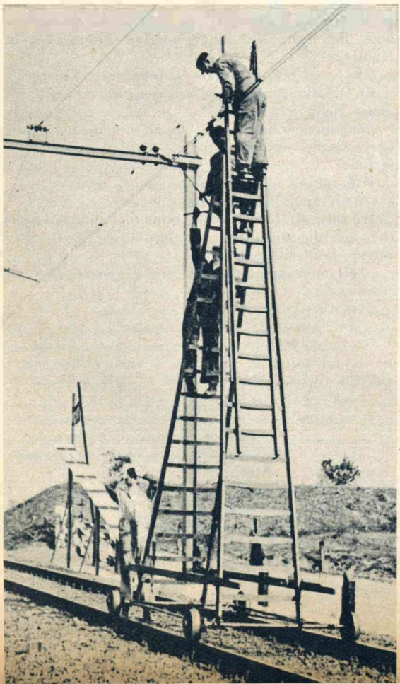
De electrische geleidingen op het traject Utrecht-Arnhem worden met spoed hersteld.
