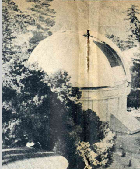
De geheimzinnige stad der sterrenkijkerij bestaat uit zilverwitte koepels.
