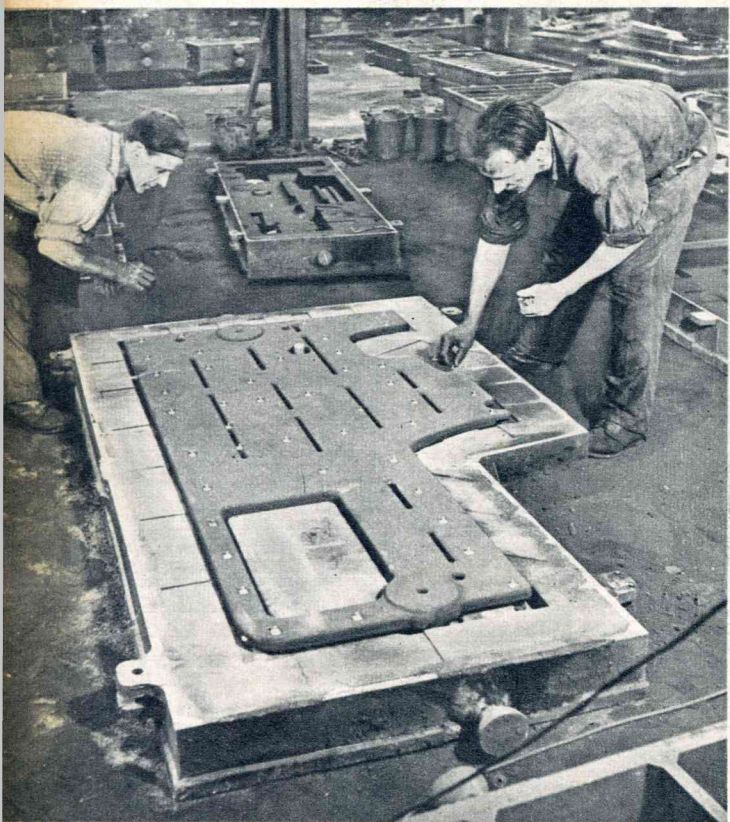
Een stuk gietijzer word uit den vorm gehaald.
