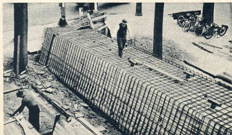
Het aantal schuilplaatsen, dat ten behoeve van de bevolking bij eventueel luchtgevaar is gebouwd, wordt nog steeds uitgebreid. Het nieuwste model dat thans vervaardigd wordt, is geheel van gewapend beton en biedt, naast grootere bescherming, ook beter weerstand aan de invloeden van ons wisselvallig klimaat.
