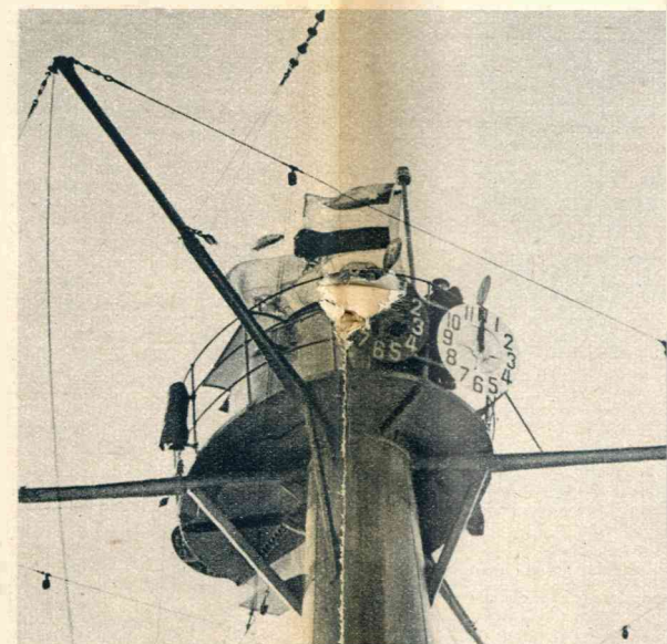
Het bovendeel van den commandotoren met ruimte voor 'n uitkijkpost. De twee wijzerplaten, die men misschien voor klokken zou houden, dienen echter om, in geval 'n storing zou optreden in de centrale vuurleiding, de hoek en den afstand van het doel kenbaar te maken aan de stuurcommandanten.
