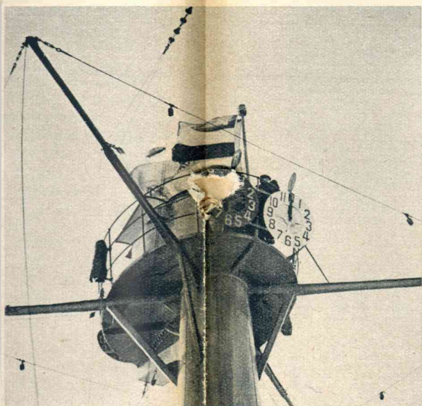
Het bovendeel van den commandotoren met ruimte voor 'n uitkijkpost. De twee wijzerplaten, die men misschien voor klokken zou houden, dienen echter om, in geval er 'n storing zou optreden in de centrale vuurleiding, den hoek en den afstand van het doel kenbaar te maken aan stukecommandanten.
