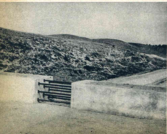
Lage betonnen muurtjes en ijzeren hekken, die zoo noodig onder stroom gezet kunnen worden, versperren de wegen in de gevaarlijke zone.
