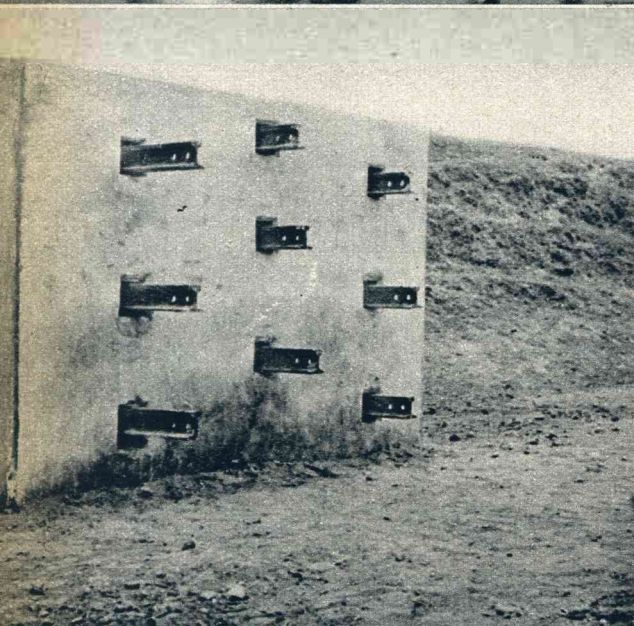
Machtige betonblokken, voorzien van ijzeren staven, staan aan de zijanten van den weg om de tanks op te houden.
