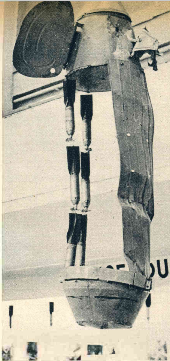
Een zoogenaamde Russische „luchttorpedo”, welke tijdens het neervallen ronddraait, zich dan in de lucht opent en een groot aantal brandbommen uitstrooit.
