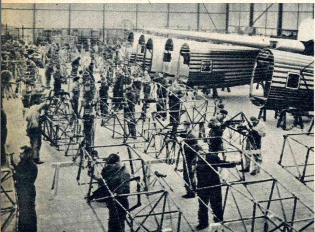
Een serie staalbuisrompen in aanbouw.
