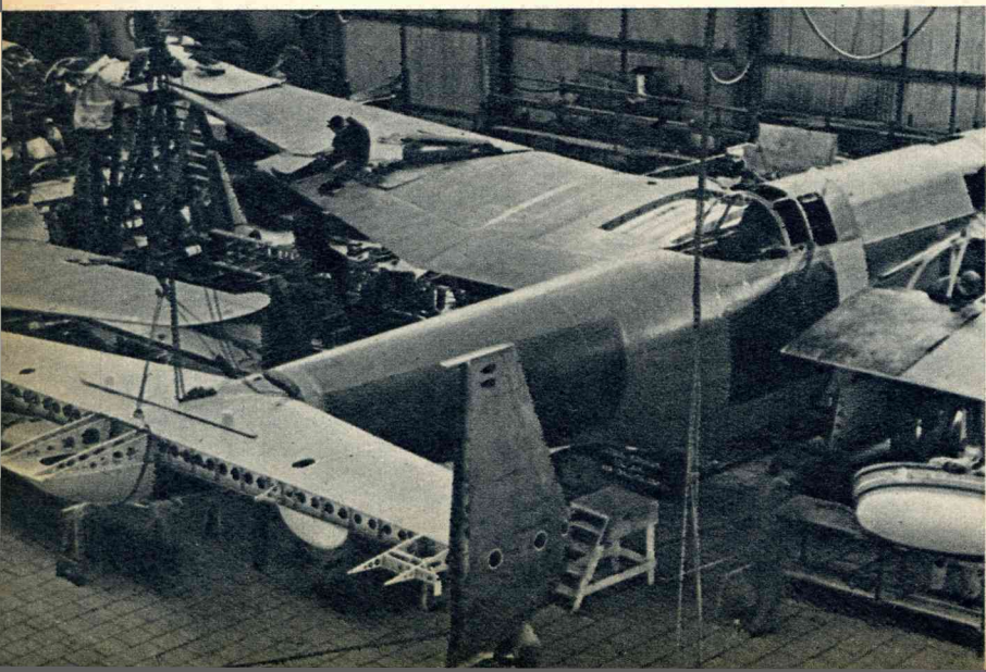
Een serie staalbuisrompen in aanbouw.
