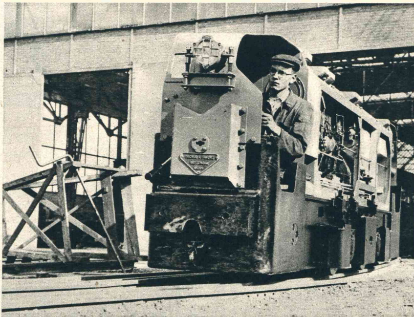
Bij de machinefabriek Du Croo en Brams te Amsterdam wordt een serie van 28 Diesel-locomotieven gebouwd, bestemd voor de ondergrondse steenkolentreinen in de Nederlandsche Staatsmijnen. Een der gereedgekomen miniatuurlocomotieven verlaat de fabriek.
