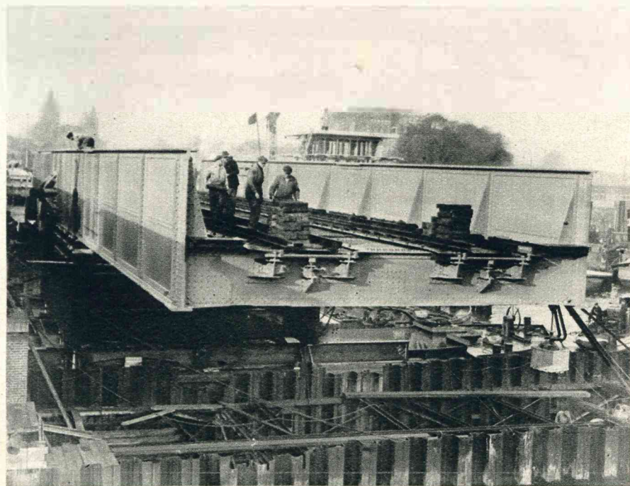
Langzaam vordert het werk voor de verbredening van den Amstelveenscheweg. Een gedeelte van de brug bij de Studionkade is nu gereed; wij naderen den tijd, dat de wegverbruikers hier niet meer in voortdurend gevaar verkeerren.
