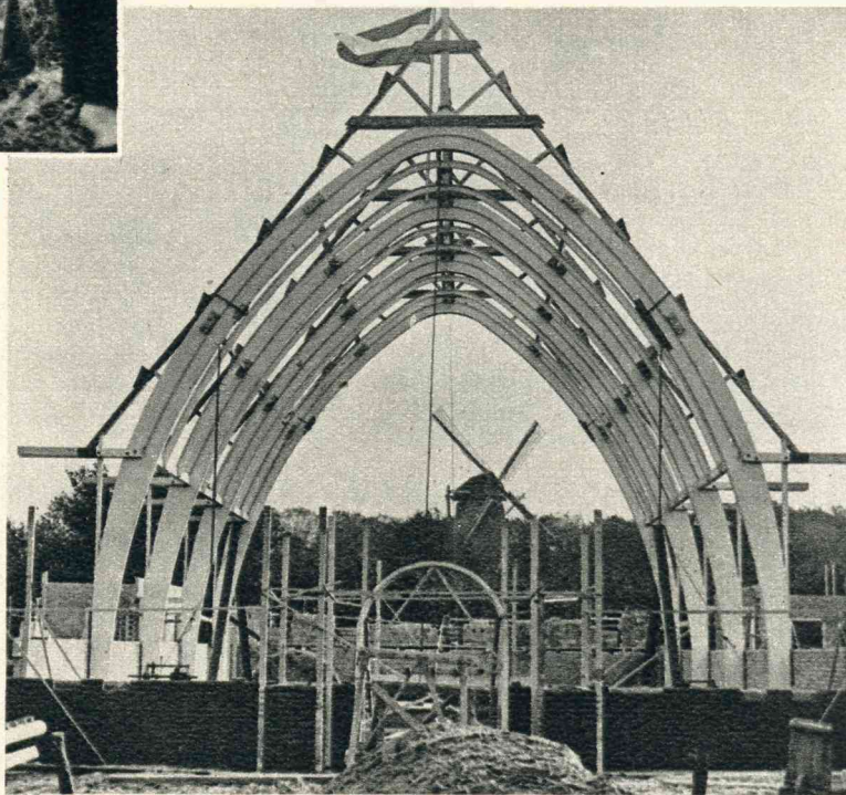
Te Santpoort wordt een nieuwe kapel der Ned. Herv. Evangelisatie gebouwd. Onze fotograaf nam een aardig overzicht van den bouw.
