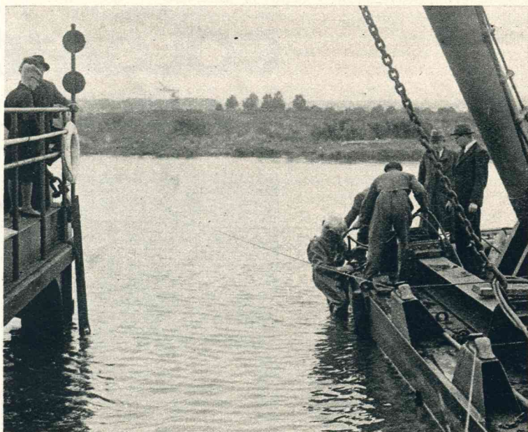
Een duiker hielp bij het moeilijke werk om de wielen van de pont op de rails te plaatsen.
