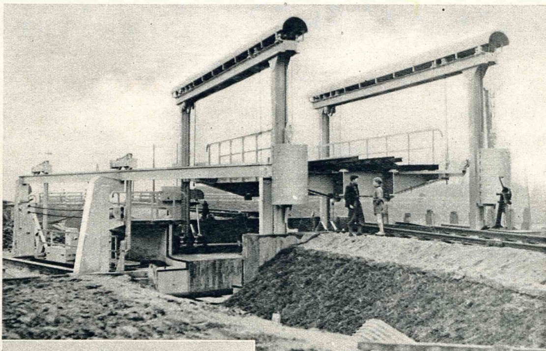
Een nieuwe spoorhefbrug is gemaakt over het kanaal Kolhorn-Alkmaar in den spoorweg, welke vanaf de groote veiling te Noord-Scharwoude naar het station van deze plaats is aangelegd.
