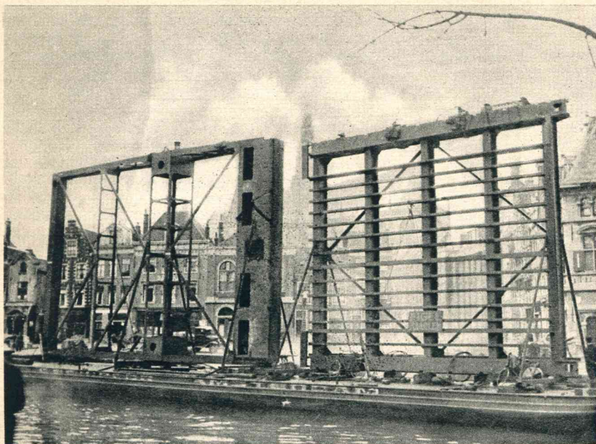
De bouw van de brug over het Zuider Buiten-Spaarne te Haarlem vordert. De ijzerconstructie voor deze brug, die een belangrijke verbetering zal brengen in het verkeer van en naar de hoofdstad, is er heen vervoerd.
