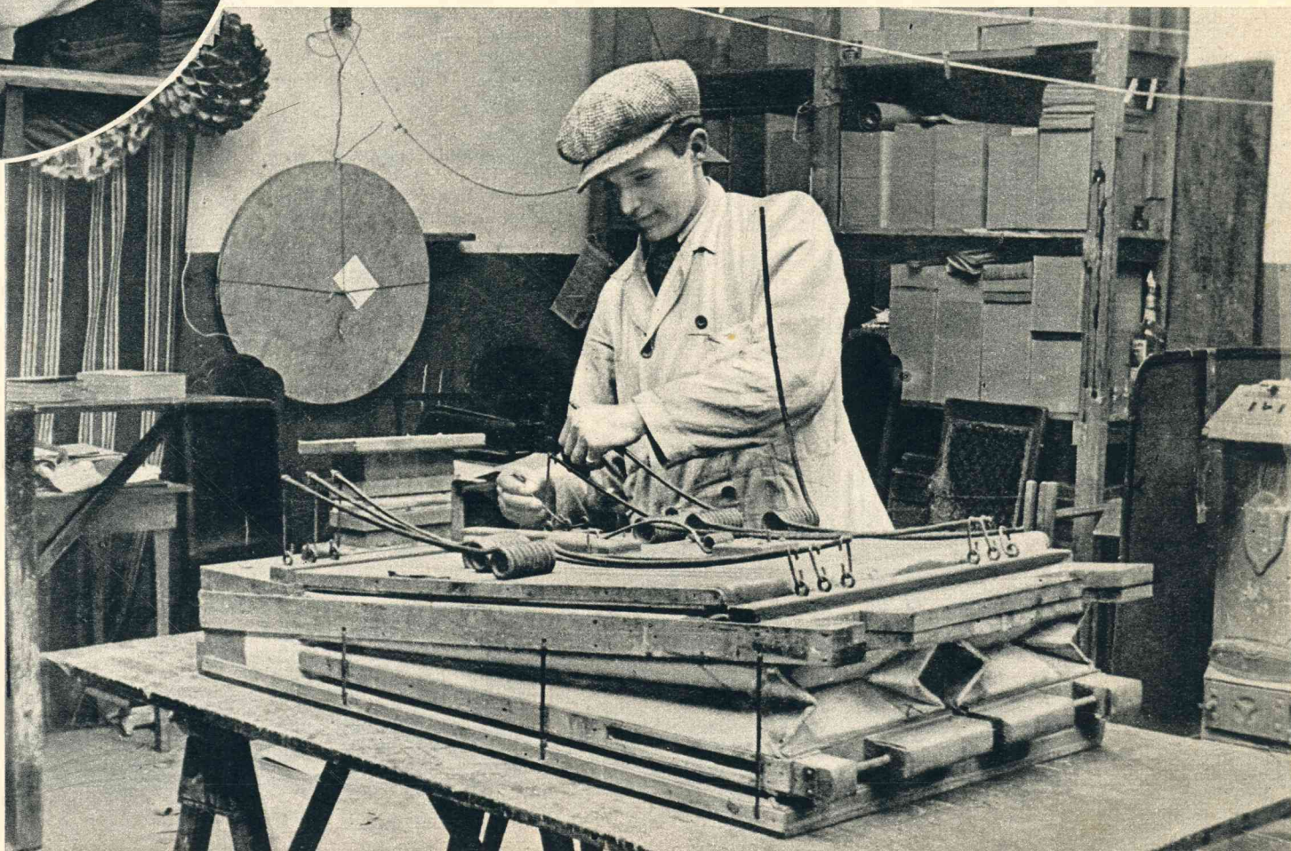
Een gedeelte van de „machine” van het pierement: windkast, windbalk, bouchettenplank en tremolo (geheel links).
