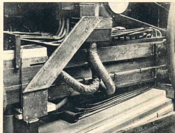
Een gedeelte van de „machine” van het pierement: windkast, windbalk, bouchettenplank en tremolo (geheel links).
