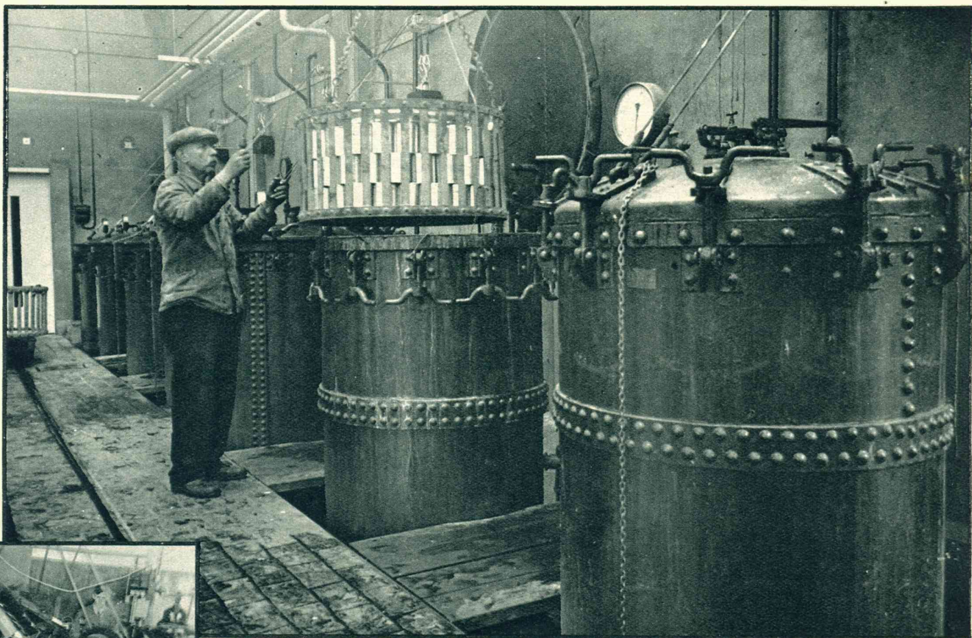
Bij groote hoeveelheden tegelijk wordt het ingeblikte vleesch in de autoclaaf geheschen.
