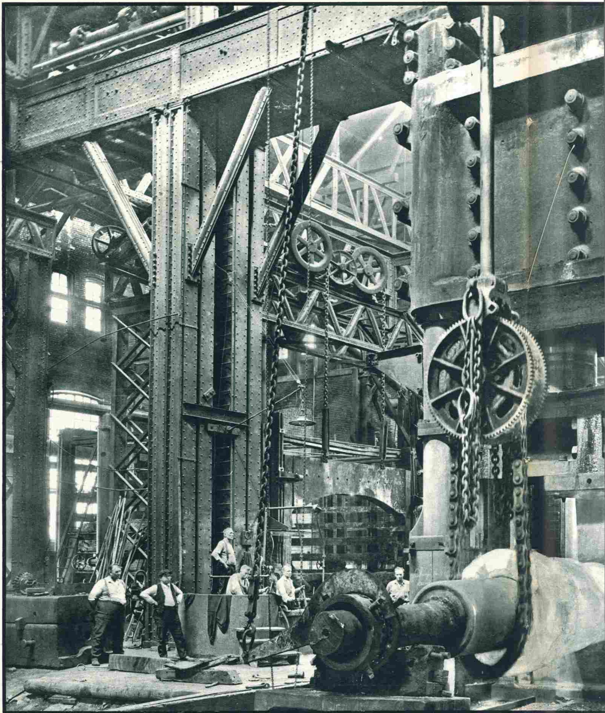
Deze enorme hydraulische smeedpers van de Bethlehem Steel Company ontwikkelt een druk van ca. 14.000.000 Kg., waarmee
