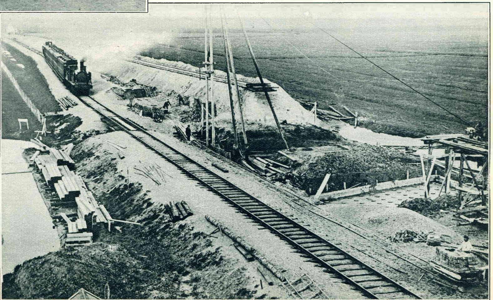
Een kijkje op de werkzaamheden aan het eerste kanaal van het West-Friesche kanalenplan, nl. de verbinding Noord-Hollandsch kanaal-Wieringer- meer nabij Scha- gen. Op de kruis- sing van de spoor- lijn Schagen-Den Helder wordt een groote draaibare spoorbruggebouwd
