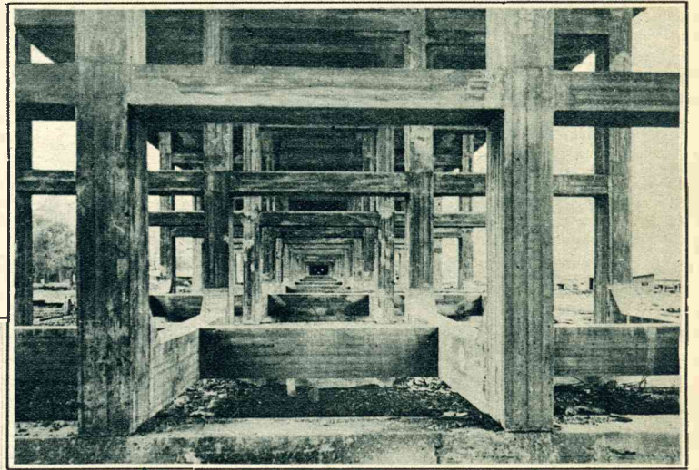
De steunpilaren van de nieuwe Merwedeburg.
