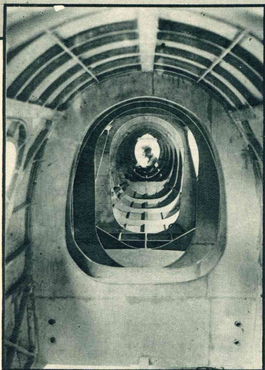
De ribbenkast van den Postjager: een kijkje van voor naar achter door den romp van het vliegtuig langs de spanten.
