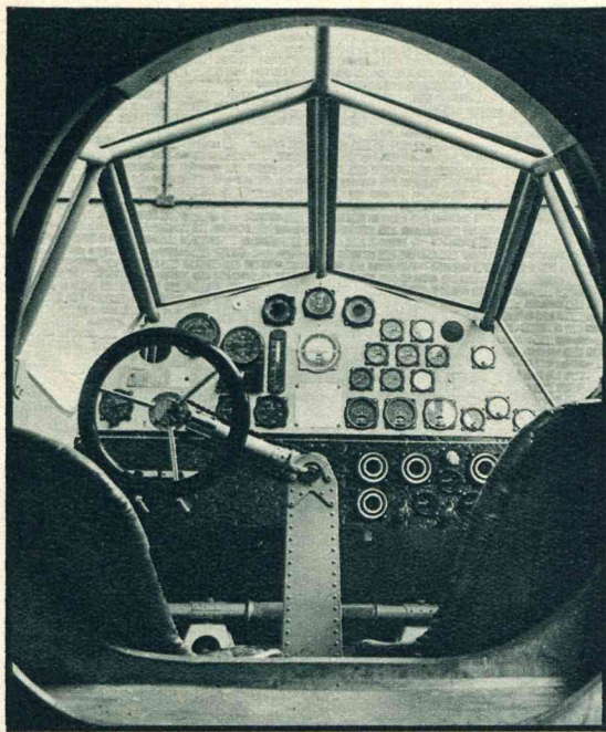
Een kijkje in de cockpit: het stuurwiel kan omgeklapt worden van den eenen naar den anderen bestuurder. De foto is genomen uit het hokje van den marconist: daarachter bevindt zich de laadruiimte voor de post.
