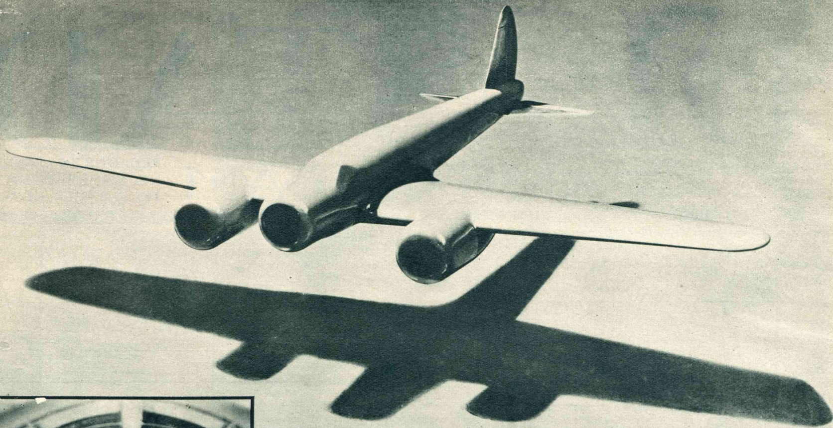
Het model van Pander's Postjager, waarmee de proeven in den windtunnel genomen zijn. Met zijn ingetrokken landingsgestel, ingekapselde motoren en gladde huid biedt het toestel den geringst mogelijken weerstand aan de lucht, waardoor de drie zware motoren een record-snelheid aan het vliegtuig moeten geven.
