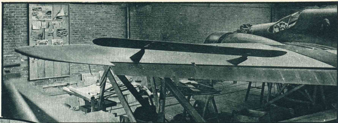
Het snelle toestel heeft een luchtrem noodig om vlot te kunnen landen. Dat is de neergeslagen flap aan den vleugel. Boven op den vleugel is de zoogenaamde aileron geplaatst, dit is het stuurvlakje waarmede het evenwicht bewaard wordt. — Deze combinatie is tot nog toe slechts in Amerika toegepast.
