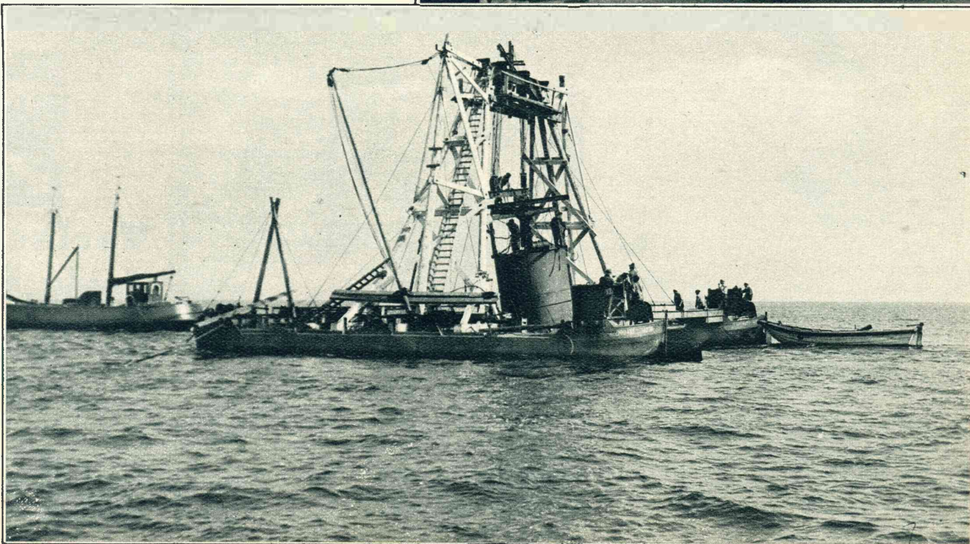
De bok is boven den vernielden toren gebracht, om den cylander er af te nemen en daarna den kegel uit het zand te trekken.
