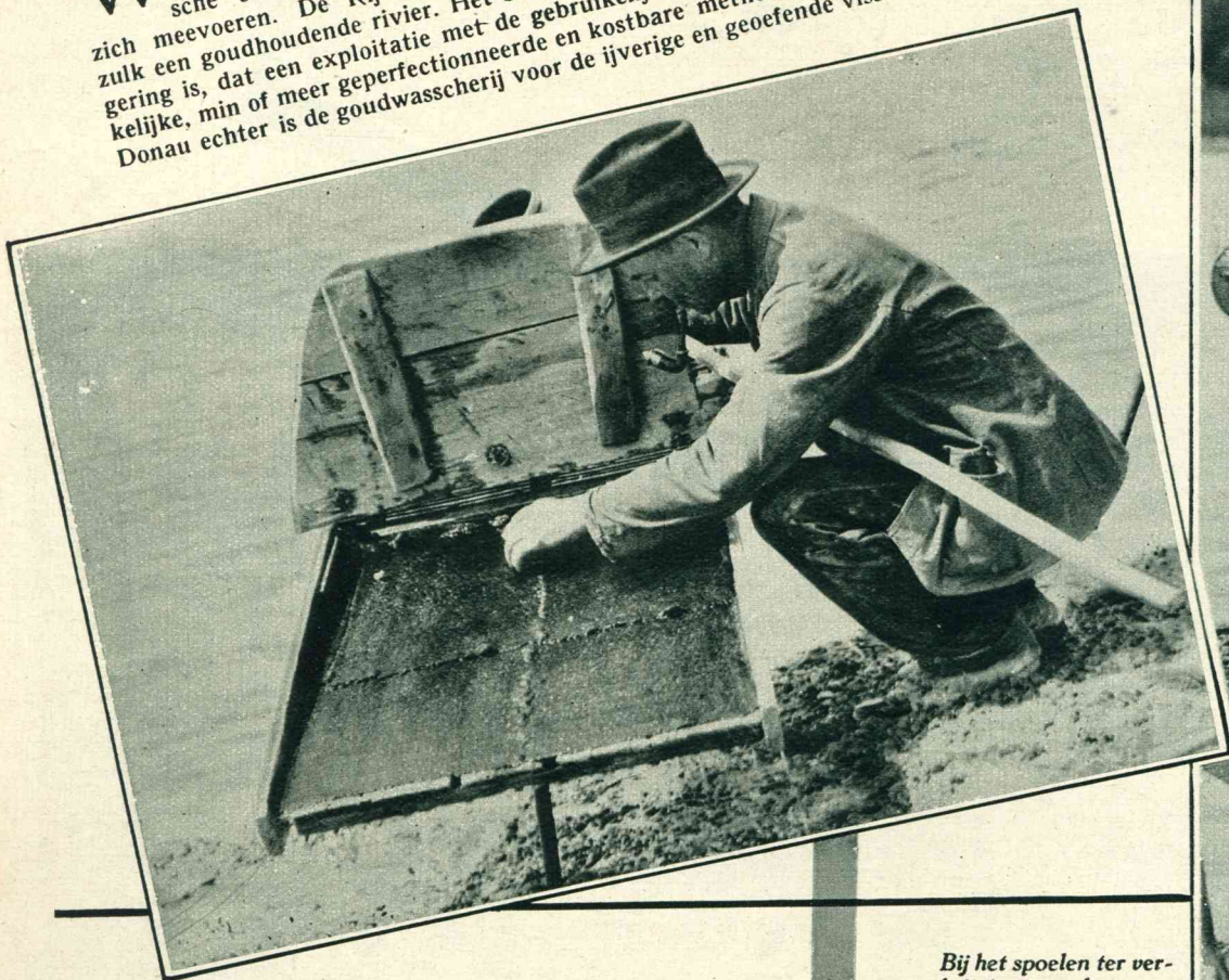
De werktuigen bij het goudwasschen zijn slechts zeer eenvoudig. Een waschapparaat, om aangespoeld goudstof te reinigen van zand, leem en andere onzuiverheden.
