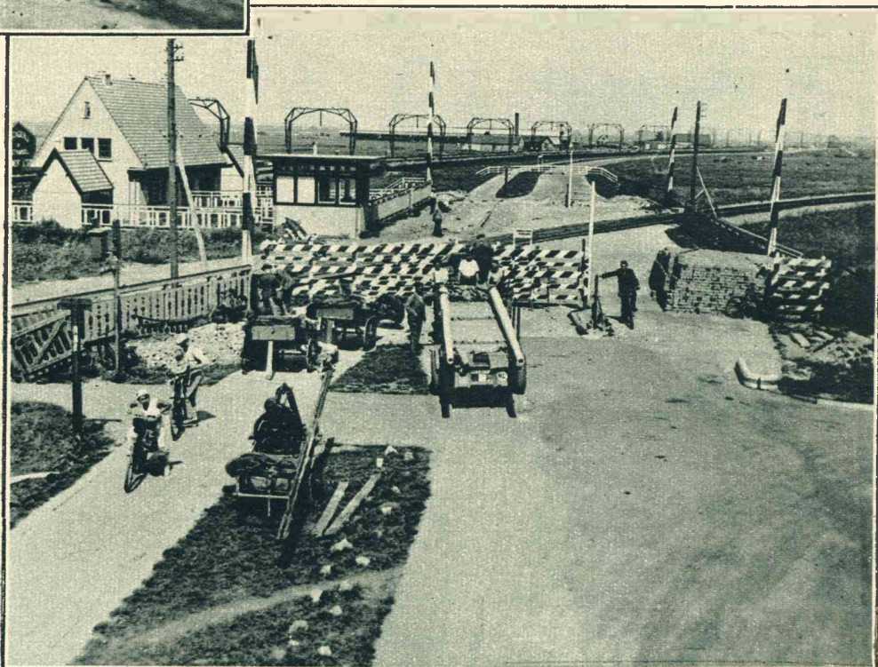
De primaire weg Amsterdam-Wormerveer is gereed gekomen. 'n Enkel obstakel moest nog worden weggeruimd, alvorens de weg definitief in gebruik kon worden genomen.
