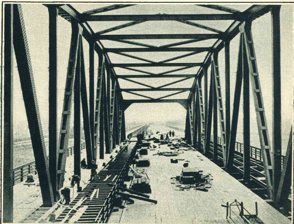
De Merwedebrug is thans geplaatst. Aan het brugdek wordt de laatste hand gelegd.
