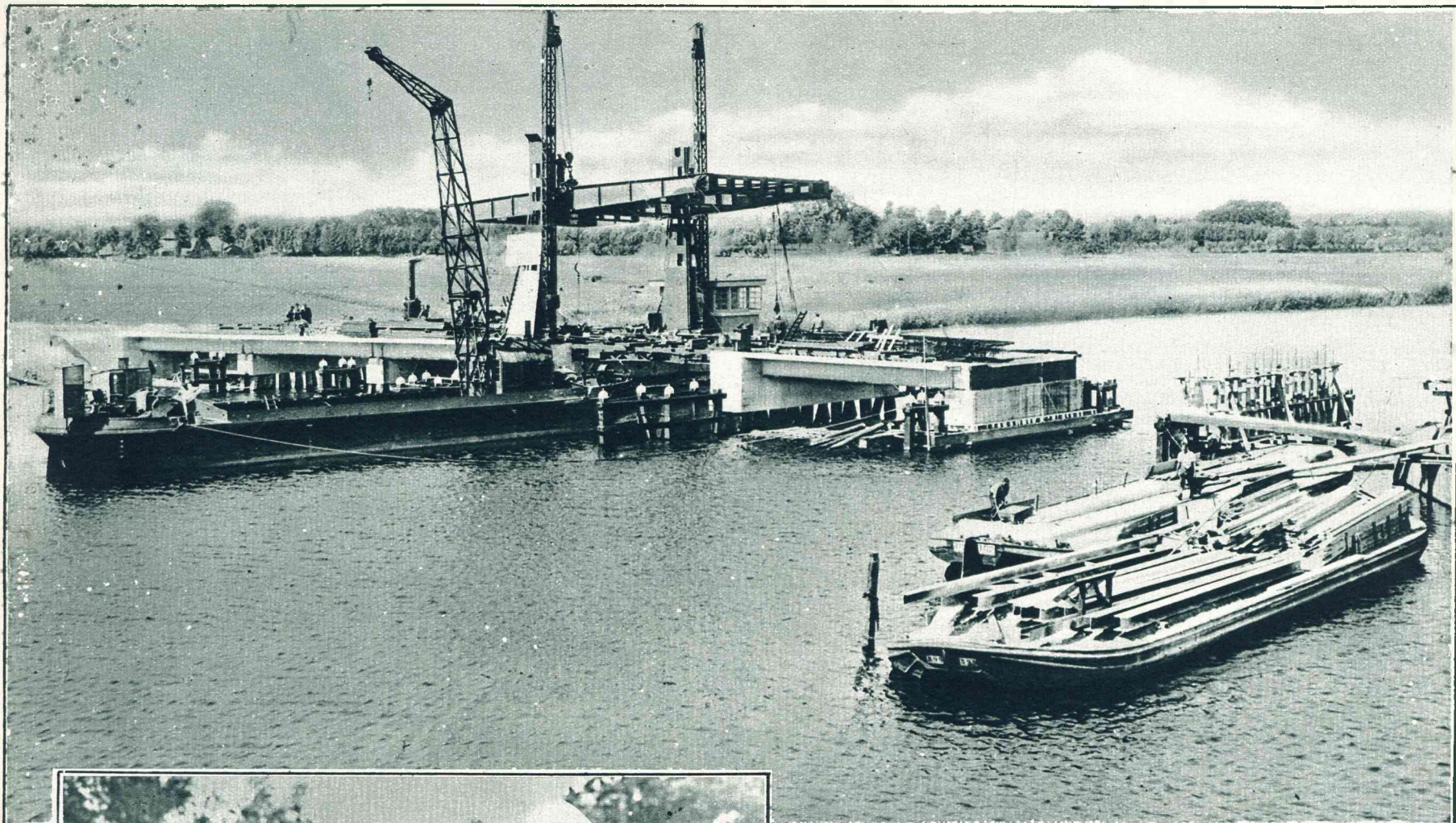
Vorige week werd de balans voor de basculebrug over de Vecht bij het fort Utermeer geplaatst. De brug ligt in den nog niet geheel gereed gekomen weg Weesp's Gravenland en heeft 'n breedte van 10 meter.
