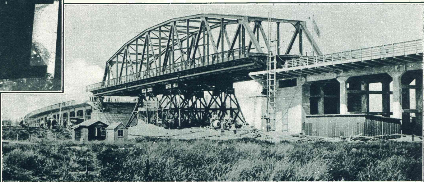
De brug over het Merwede-kanaal is geplaatst. Een overzicht van het nieuwe viaduct aan den Muiderstraatweg, toen de brugboog tusschen de landhoofden was gearriveerd en nog niet op de pijlers rustte.
