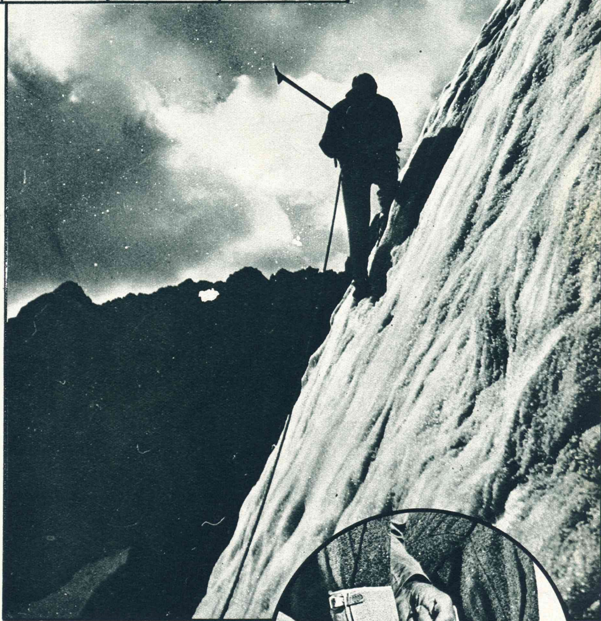
Meer dan zeventig graden helt de opgestuwde ijsmassa.
