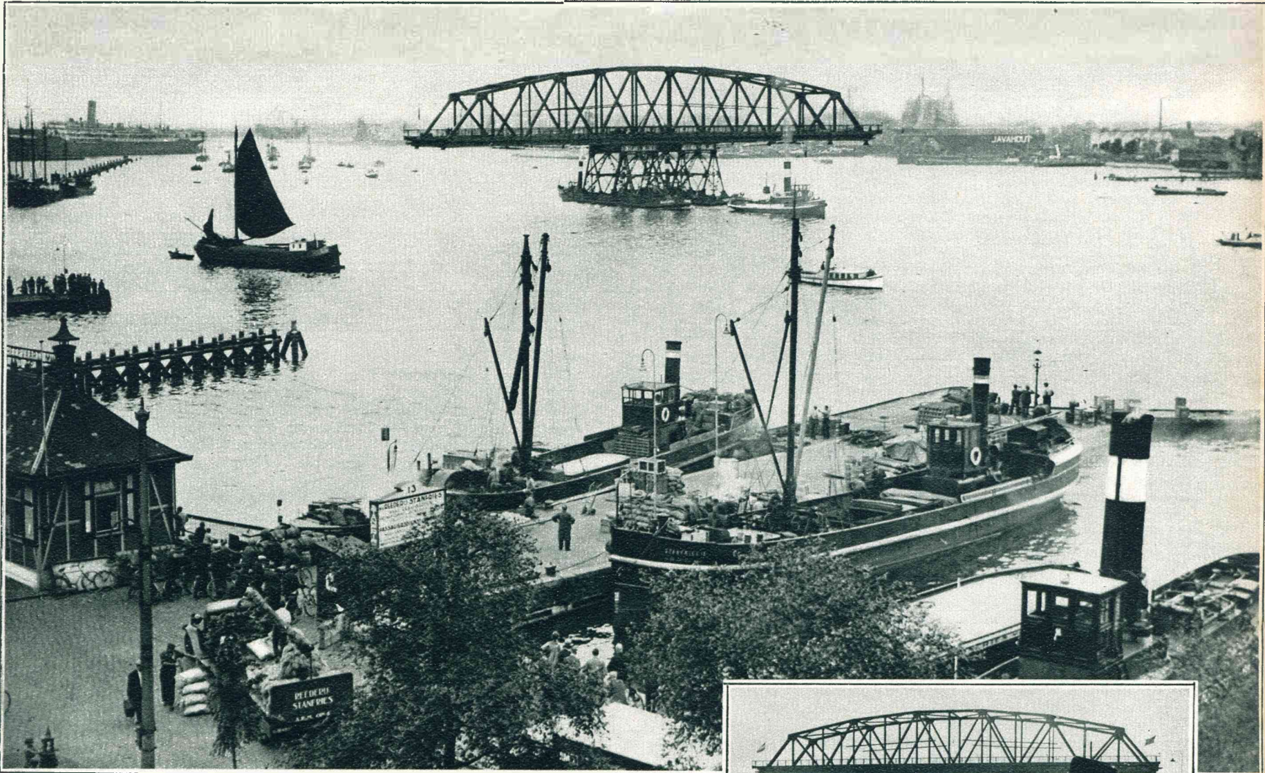
Na het verlaten van de werf der Ned. Dok Maatschappij werd de brug over het IJ gesleept. Het transport.
