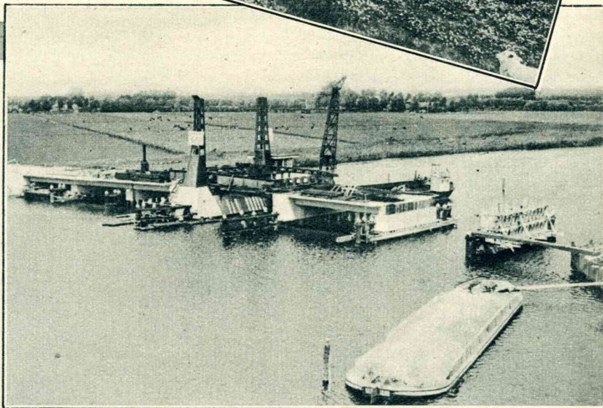
Voor den tweeden grooten verbindingsweg van Amsterdam naar het Gooi, welke voor een deel langs het tot primairen weg omgebouwde Weesperzandpaa zal loopen, wordt thans bij fort Uittermeer een brug over de Vecht gebouwd. De brug zal geheel uit beton worden gebouwd, krijgt een lengte van 100 M. en een breedte van 10 M.
