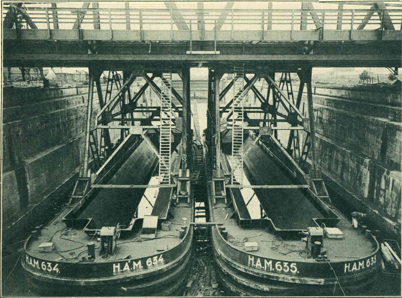
De beide pontons waarop de nieuwe Merwede brug rust en die het gevaarte uit het dok van de Ned. Dok Maatschappij naar de plaats van bestemming zullen vervoeren.
