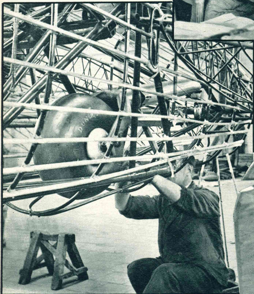
Het construeeren van het staartwiel, dat in den romp van het vliegtuig kan worden getrokken.
