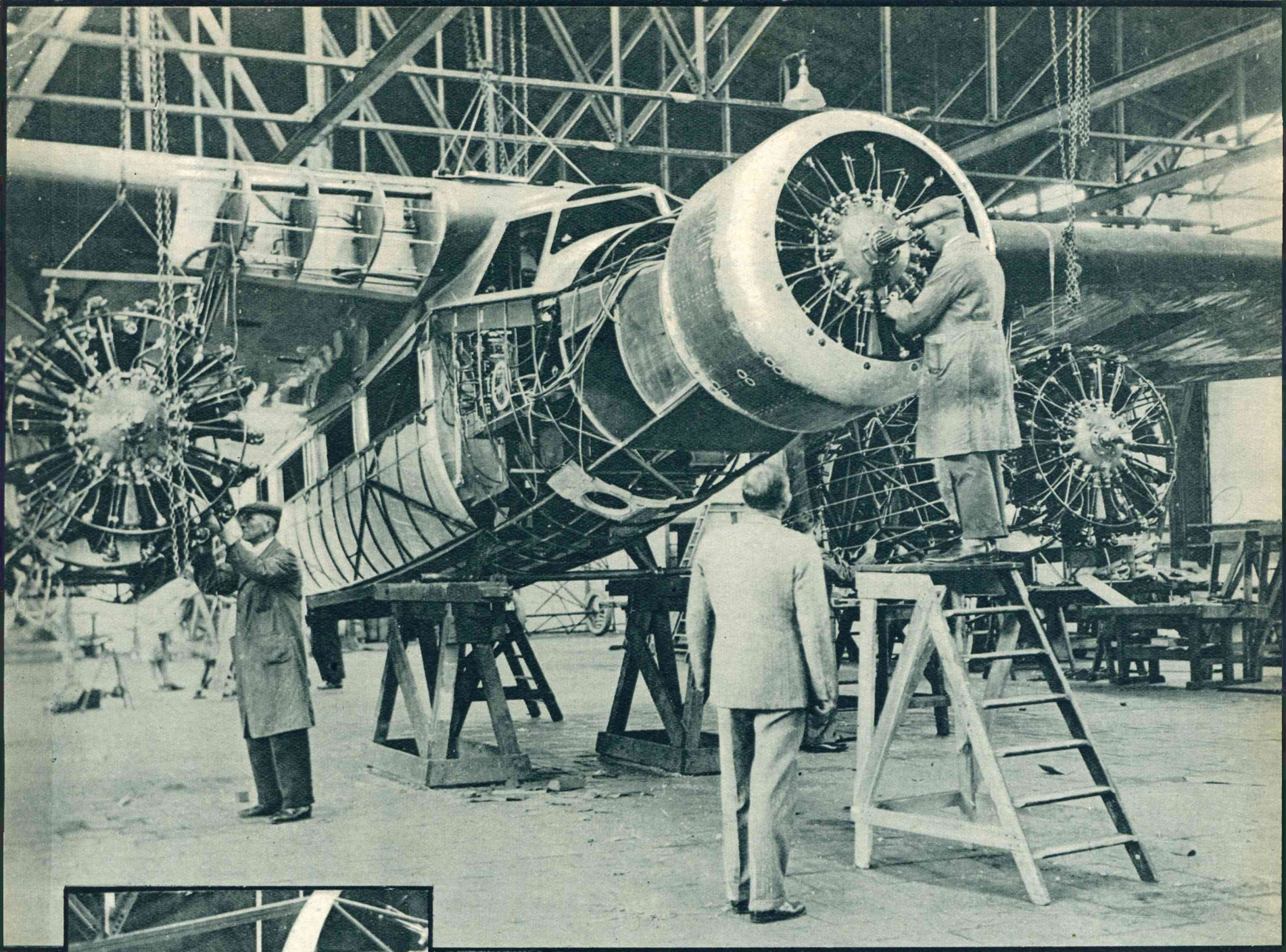
Het plaatsen der motoren in de F.XX.
