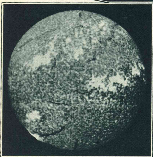
Opname der zon met den spectroscop in het licht der calciumlijn met lichtende protuberansen en donkere calcium-wolken.
