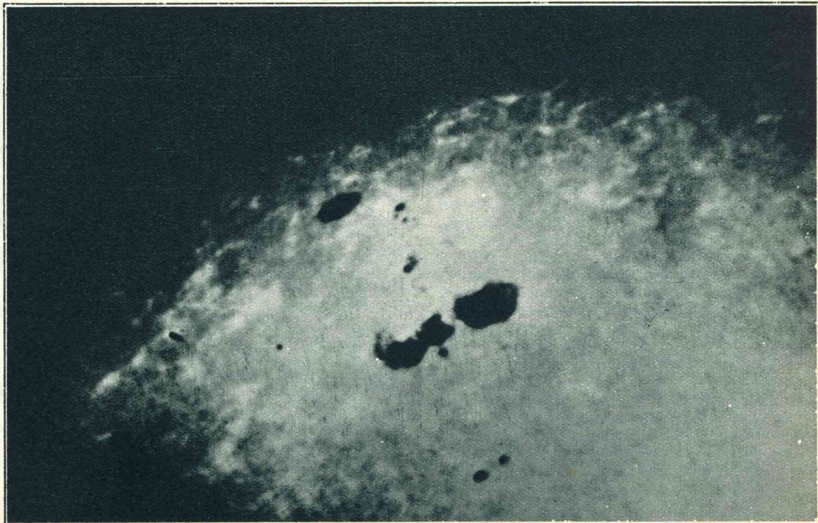
Groep zonnevlekken temidden van uitgebreide fakkels.
