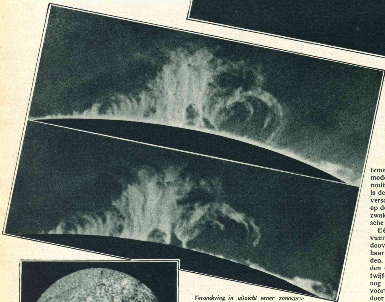
Geweldige protuberansen worden tot 150.000 K.M. in het wereldruim geslingerd.
