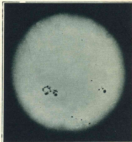
Zonnesfoto met groote plekkengroepen en fakkels.
