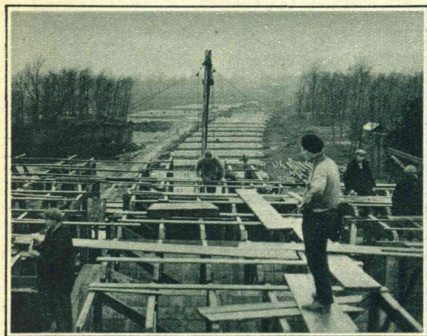
De nieuwe brug aan den Muiderstraatweg, over 't Merwedekanaal, wordt eveneens goed. De aanleg van den oprit.
