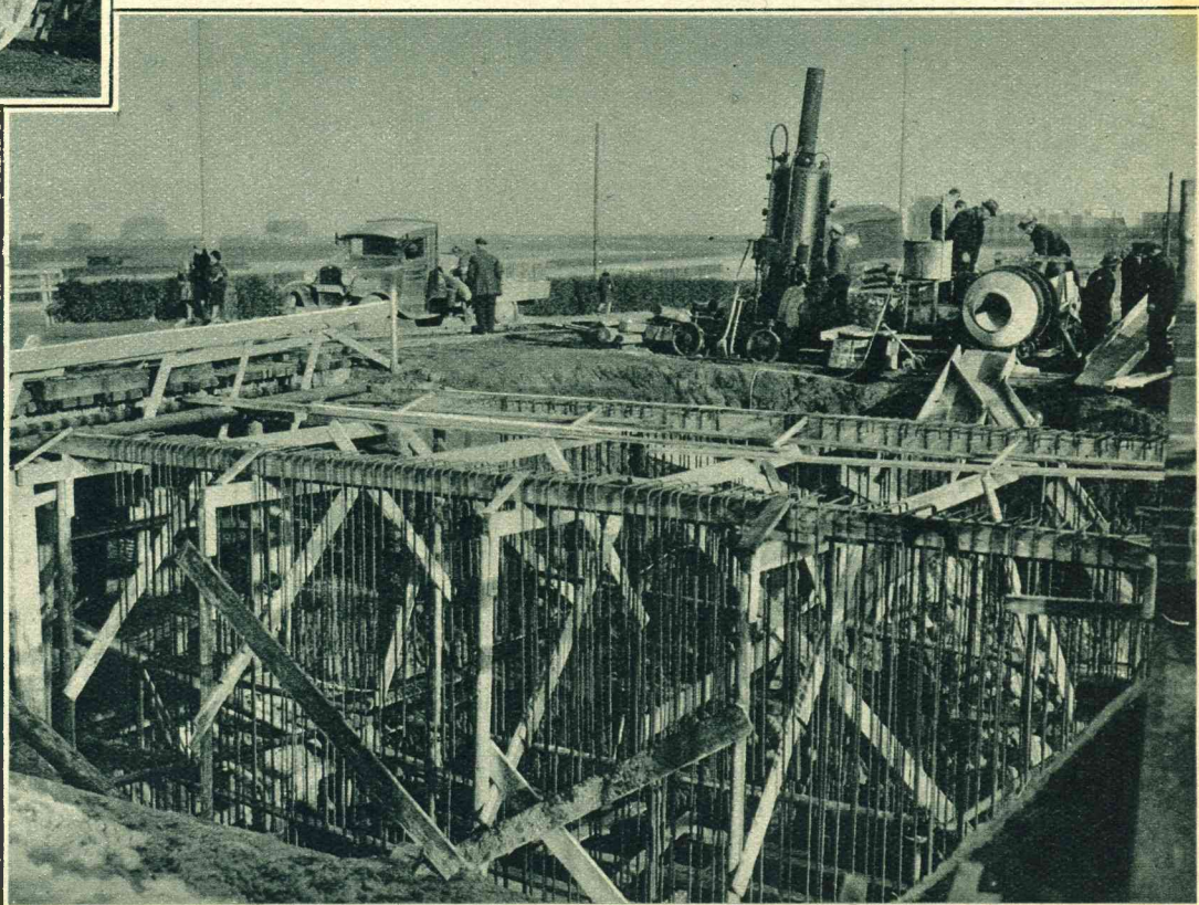
In den Rijksweg van Haarlem naar Sassenheim wordt de oude Lisserbrug vervangen door een duikerbrug. De werkzaamheden zijn in vollen gang.
