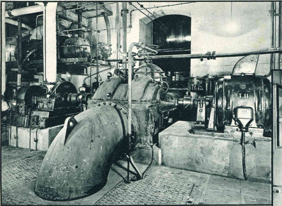
De afgewerkte stoom der turbines wordt weder tot water gecondenseerd in twee condensors. Het hiertoe benodigde water wordt opgebracht door de hier afgebeelde pompengroepen.
