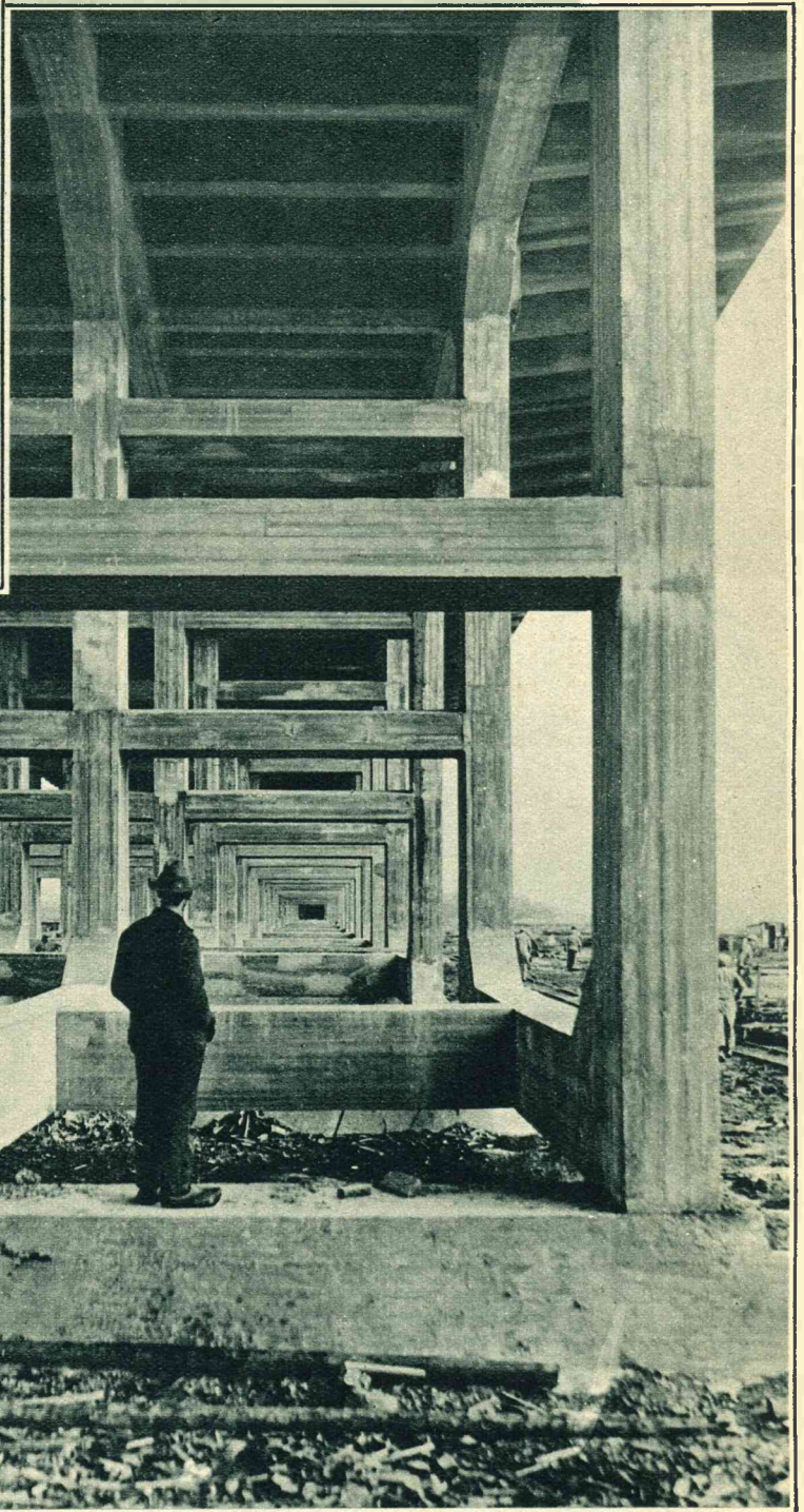
De laatste betonstorting in het Oostelijk gedeelte van de in aanbouw zijnde brug over het Mervedekanaal is geschied. Een doorkijkje onder de brug.
