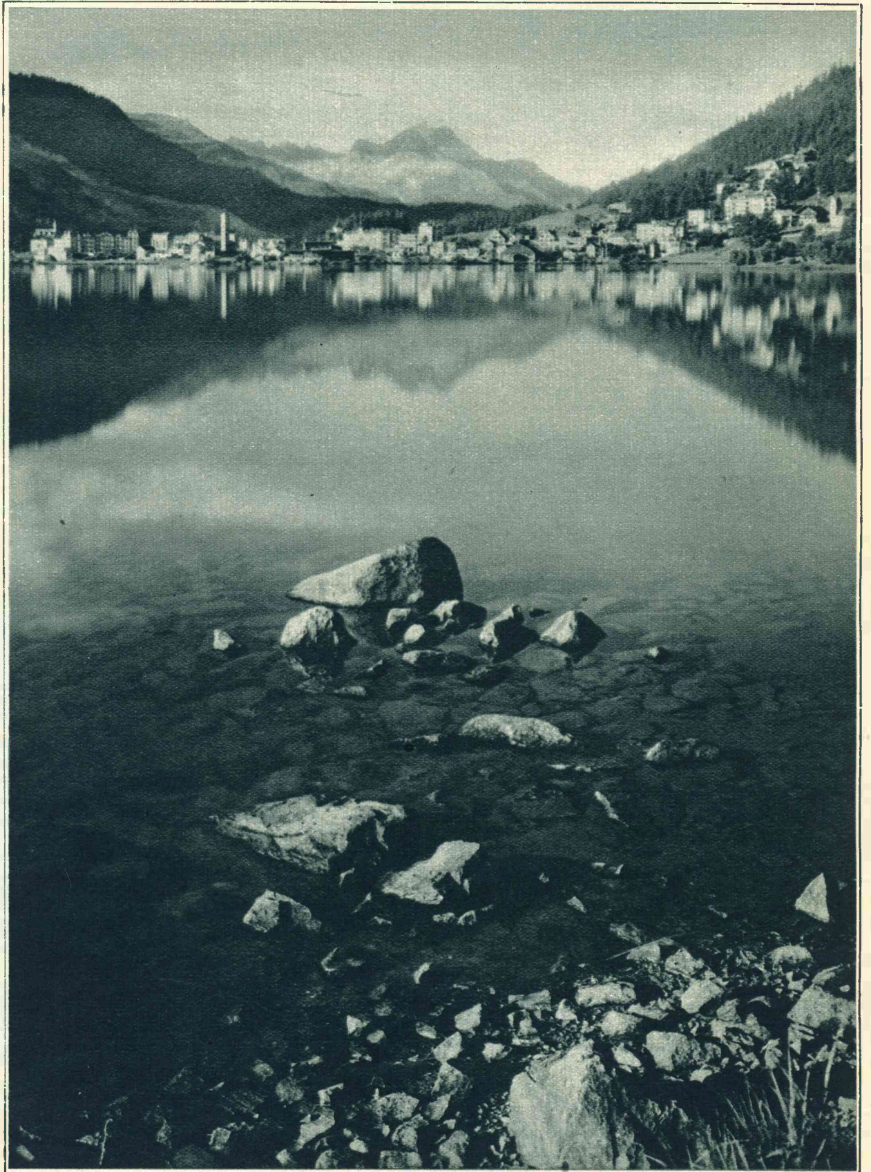
Zoo helder is onder de blaauwe luchten 't water in de St. Moritzersee, dat men er de steenen op den bodem tellen kan.
