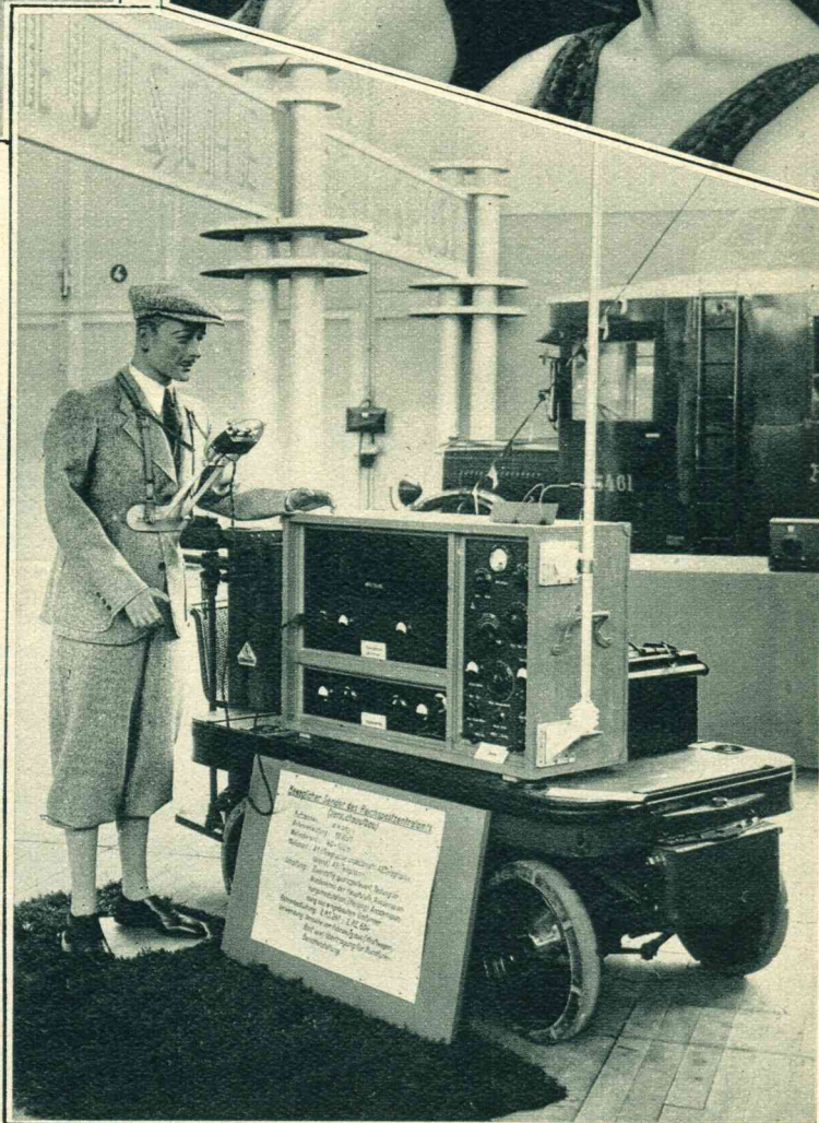
Van de Berlijnsche Radio-tentoonstelling. — Veel belangstelling trok de verplaatsbare zender van de Rijkspostcentrale. — Hij wordt bewaakt door een nagemaakten mensch
