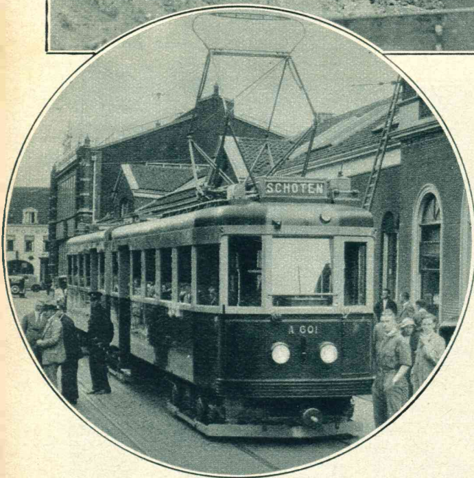
Met den eersten der serie van 10 nieuwe harmonica-wagens, door de fa. Beynes aan de N. Z. Holl. Tramwegmij. geleverd, werd begin dezer week te Haarlem proefgereden. Er was veel belangstelling voor den fraaie tramwagen.
