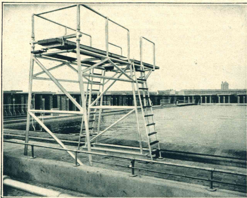
De soepel geconstrueerde springtoren.
