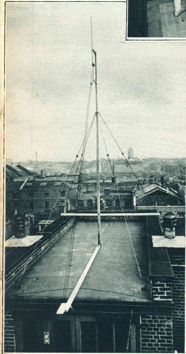
De speciale antenne, welke door de Baird Television Comp. te Londen is opgericht op het dak van haar laboratorium ten behoeve van de experimenten op ultra-korte golven.
