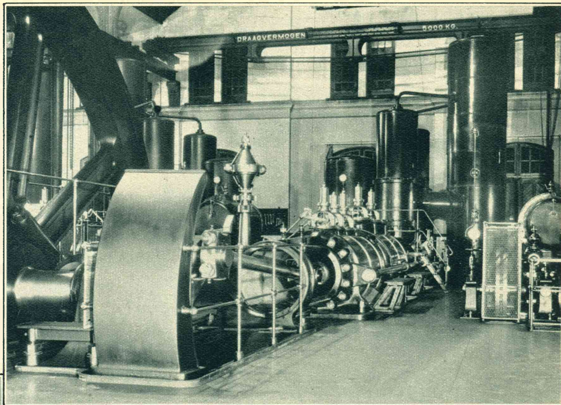
Interieur van de machinekamer van het pompstation aan den Haarlemmerweg te Amsterdam.
