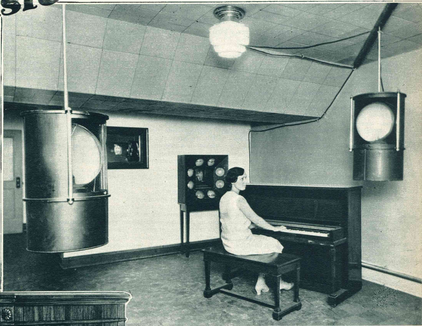
De studio van het Amerikaansche Televisie-station van de National Broadcasting Comp. Inc. te Chicago. Tegen den muur staat op een tafeltje de kast met de batterij foto-electrische cellen, die tot taak hebben de lichtvariaties om te zetten in elektrische trillingen, welke via versterkers en zenders worden uitgezonden.
