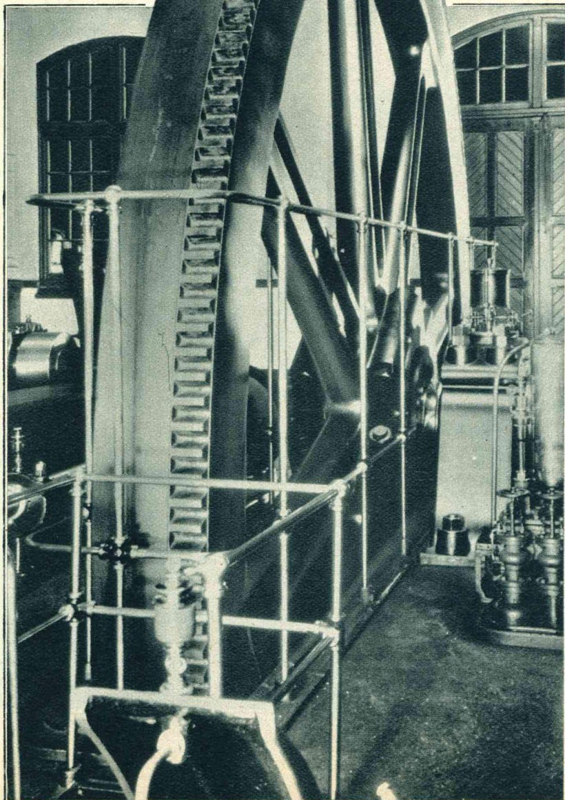
Het reusachtige vliegwiel in het pompstation aan den Haarlemmerweg.
