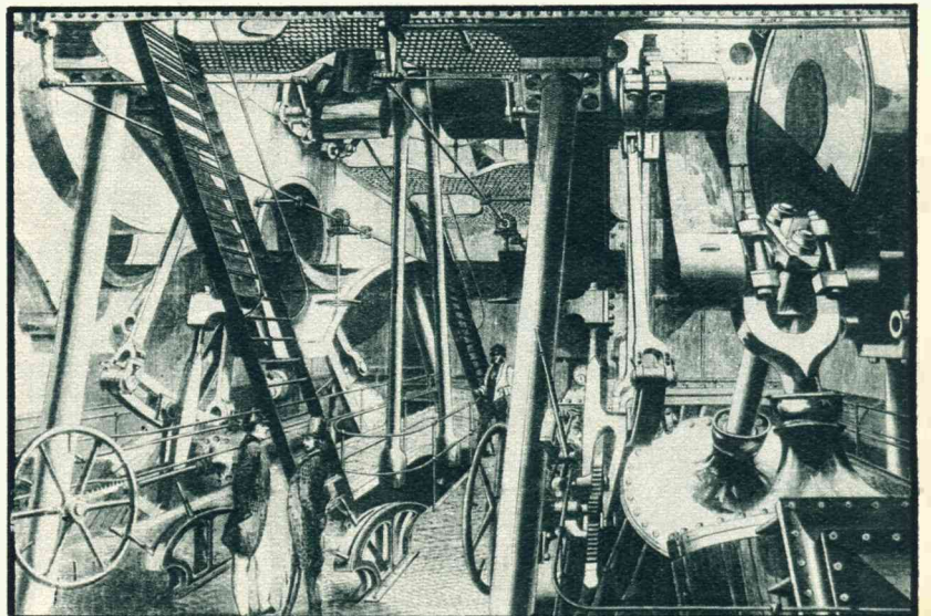
De machinekamer van de „Great Eastern”, die 207 lang was, en waarin alle tijdgenooten van verbazing niets anders konden doen dan zwijgend bewonderen.
