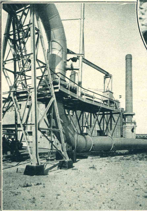
De centrale van de P.E.N.: op den voorgrond de reusachtige gastoevoerbuis naar de hoogovens.
