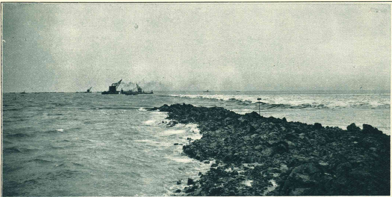
Het laatste gat in den dijk, zooals er dat voor enkele dagen nog was en waar toen bij vloed en bij eb het water nog met groot geweld in- en uitstroomde. Duidelijk was, en is ook op de foto, het verschil in waterstand te zien.
