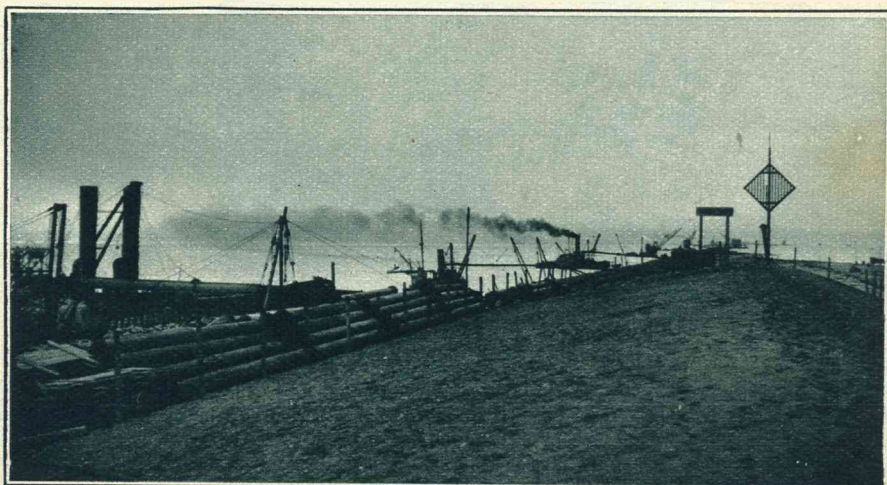
Een kijkje op den dijk, dicht bij De Vlieter, waar nog druk gewerkt wordt.
