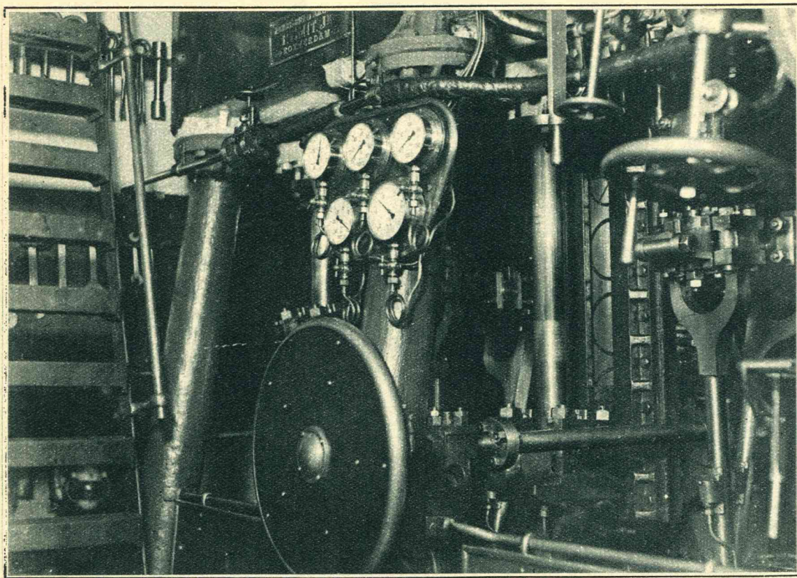
De machinekamer van een IJmuider trawler.
