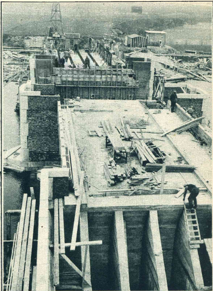
Ten behoeve van den nieuw aan te leggen weg Amsterdam-Velsen wordt een groote verkeersbrug gebouwd over het zijkanaal F.
