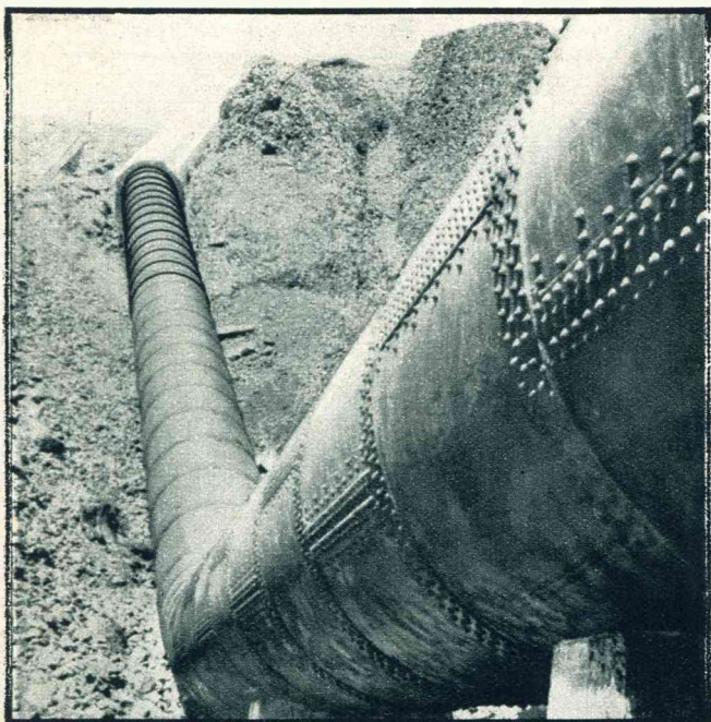
Over woeste bergruggen wordt, zooals hier in den staat Washington (Yakima-district) het water door geweldige buisleidingen gedreven (binnenwijdte drie à vier meter) naar streken, die anders van 't levenwekkend vocht verstoken moeten blijven.
