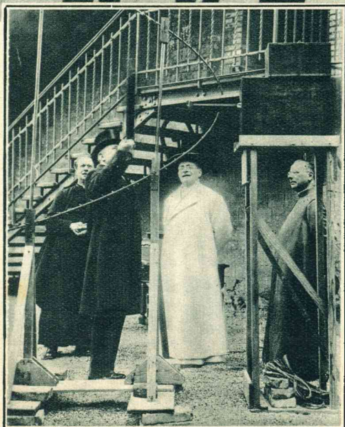
Paus Pius XI bezichtigde de korte-golf-installatie, welke door Marconi in het Vaticaan is gebouwd en welke met het Pauselijk zomerverblijf Castalgandolfo zal worden verbonden.
