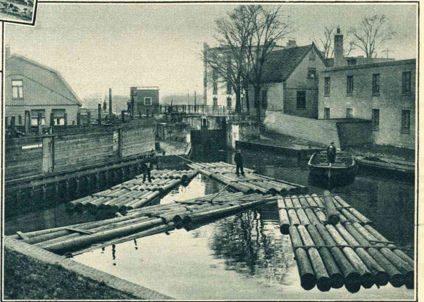
De Jaaphaversluis te Zaandam vormt een ernstige belemmering voor de binnenscheepvaart. Hoewel de gelden voor een verbeterde doorvaart reeds lang zijn toegestaan, verkeert alles nog in denzelfden toestand.
