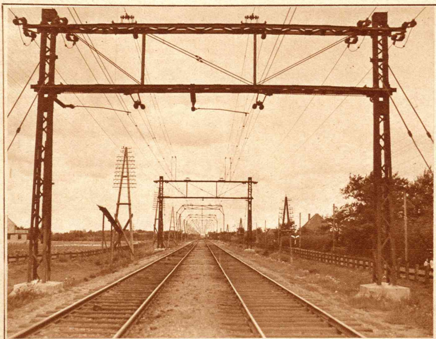
De electricificatie van de spoorlijn Amsterdam— Alkmaar vordert thans snel, zooals onze foto bewijst.
