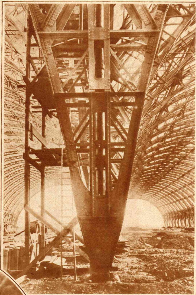
Binnenkort zal het nieuwe stations-gebouw van Milaan voltooid zijn. Een foto van de geweldige overkapping, die de perrons zal omspannen.
