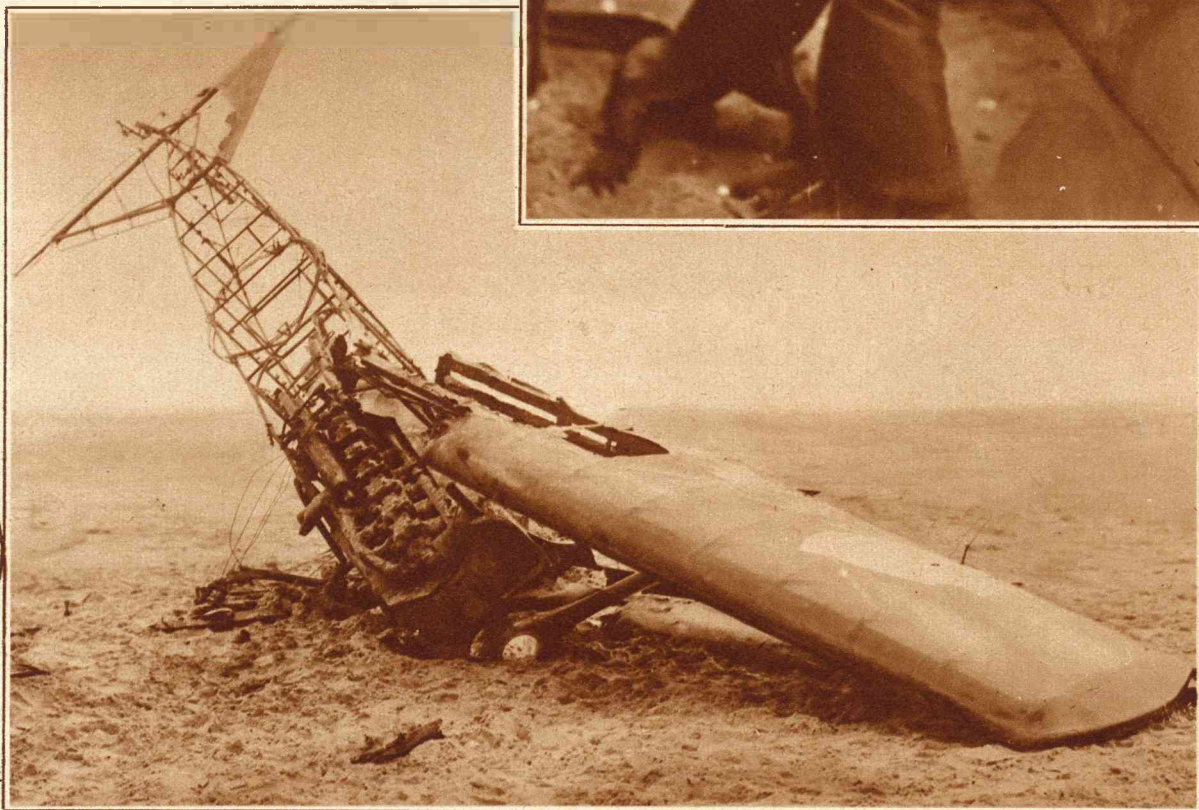
Het militaire vliegtuig C.I no. 508, gedetacheerd bij het Vlieggkamp de Kooy, moest op de Zandplaats Onrust bij Texel een noodlanding maken, waarbij het in brand vloog en totaal verminkt werd. De vliegers, serg. Mutsaers en Siebema, werden gewond naar het hospitaal te Den Helder overgebracht.
