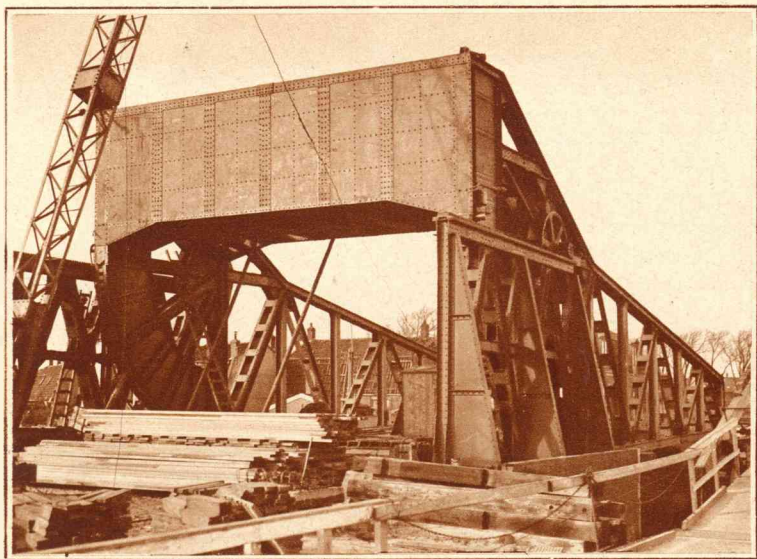
Een kijkje op de werkzaamheden aan de nieuwe brug over 't Bassin te Den Helder.
