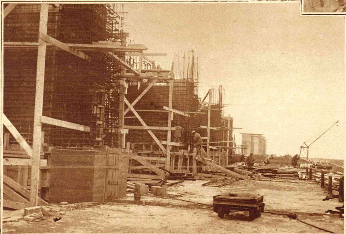
BOVEN OP DE UITWATERINGSSLUZEN — Aan deze zijde komt de weg voor het gewone verkeer. We zien hier tevens de bewapening van de heftorens.
