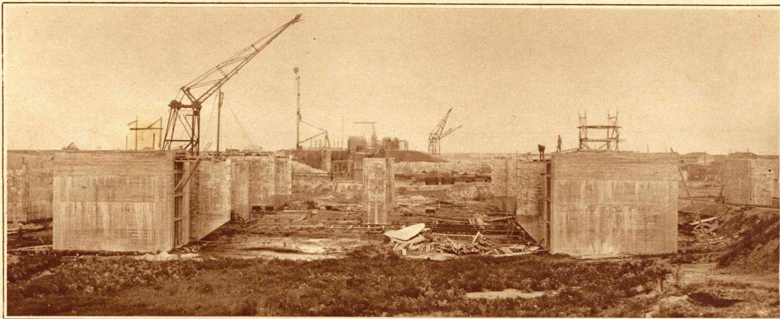
WAAR DE VERBINDINGSWEG HOLLAND—FRIESLAND KOMT — Op den voorgrond de pijlers van de spoorbrug (links) en de verkeersbrug (rechts). In 't midden daarvan de pijlers, waar bij open stand van de brug deze op komt te rusten. Achteraan zien we de heftorens van de uitwateringssluizen.
