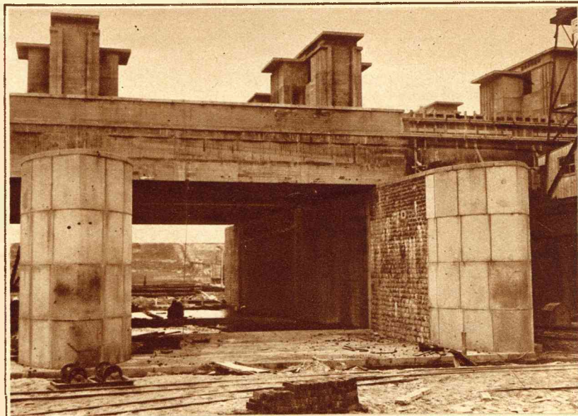
EEN COMPLEX VAN 5 UITWATERINGSSLUIZEN — De uitwateringssluizen zijn gereed. Met den bouw van den heftorens is men nog druk bezig.
