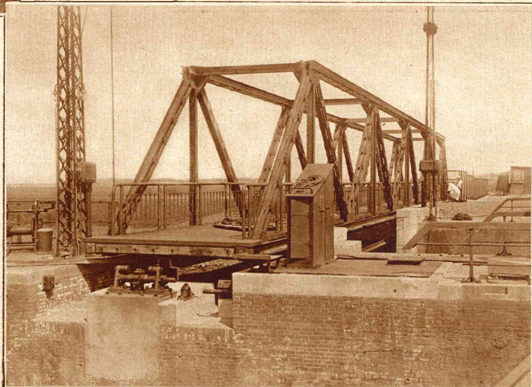
IN IJMUIDEN. — Doordat er waarschijnlijk een constructiefout heeft plaats gehad, wil de rolbrug bij de Oude Sluis te IJmuiden niet functionneeren, hetgeen natuurlijk zeer veel last veroorzaakt.
