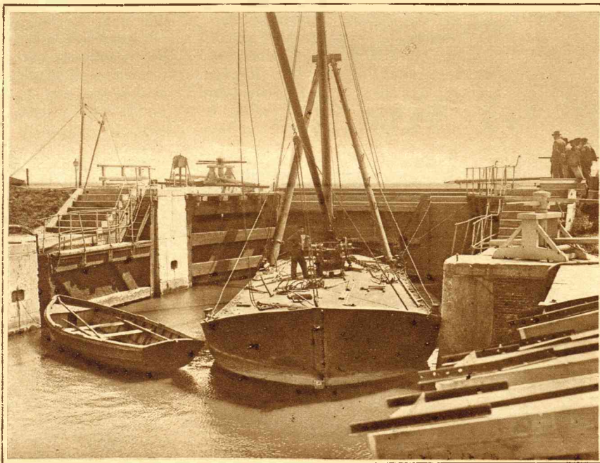
De sluis te Enkhuizen zal gerepareerd worden. Met de werkzaamheden der voorbereiding, n.l. het vervangen der deuren door waterdichte schotten, is, zooals men op onze foto ziet, reeds een aanvang gemaakt.
