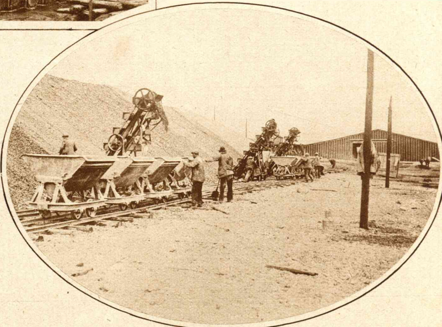
Een detail. Een kijkje op de grint-voorraden voor de vervaardiging der betonspecie.
