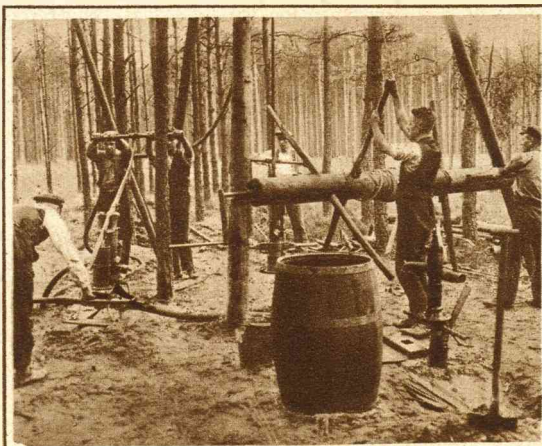
In de bosschen van Erkner, in de nabijheid van Berlijn, worden boringen naar bruinkolen gedaan.
