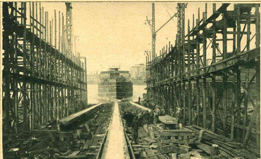
De te waterlating van de „Julieta" van de werf der Ned. Scheepsbouw Mij. De Julieta is een stalen tankschip van \pm 2300 tons dat voor Engelsche rekening gebouwd werd. Het schip verlaat de werf.
