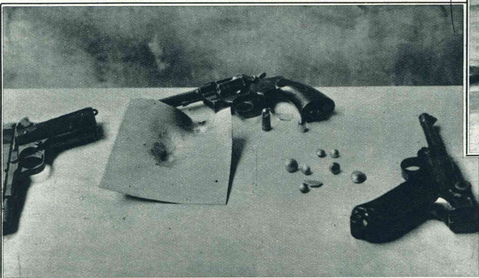
De moord op koning Alexander en minister Barthou te Marseille heeft een Fransch politiebeambte tot de samenstelling van een nieuwe pantserstof gebracht, half metaal en half rubber. Zooals men ziet werd deze stof door kogels van verschillend kaliber niet doorboord, alleen ingedeukt.
